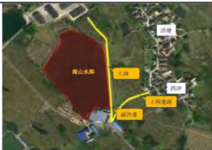
南山水库现状及本项目改造范围
